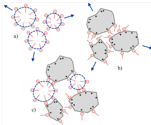
Rysunek 1. Podstawowe mechanizmy działania domieszki napowietrzającej BETOCEL 5A (opis w tekście)
